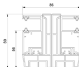
Delad PVC-styrskena - RS, inspektionsslucka från utsidan. MK933 + MK9730
