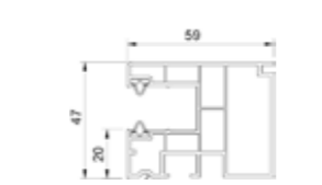
Ensidig PVC-styrskena - RS, inspektionsslucka från insidan. MKM928(7)
