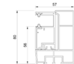
Ensidig PVC-styrskena - RS, inspektionsslucka från utsidan. MK933 + MK9760
