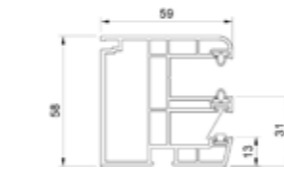
Ensidig PVC-styrskena + MKT* - RS, inspektionsslucka från insidan. MK8110
