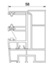
Ensidig PVC-styrskena + MKT* - RS, inspektionsslucka från utsidan. MK8120 + MK9760
