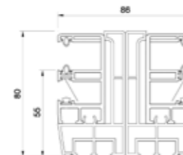
Delad PVC-styrskena + MKT* - RS, inspektionsslucka från utsidan. MK8120 + MK9730
