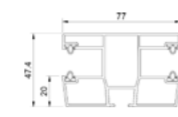
Delad PVC-styrskena - RS, inspektionsslucka från insidan. MK939
