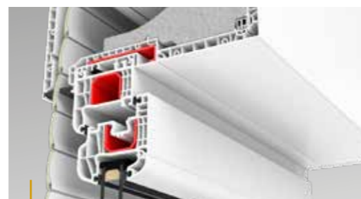
Adapter för Iglo 5.
