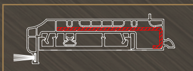
förstärkt adapter
