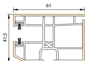
enkel styrskena
